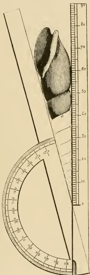
Fig. 267. D'Orbigny's Helicometer.
